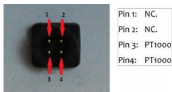
Rysunek 22.1 Złącze
